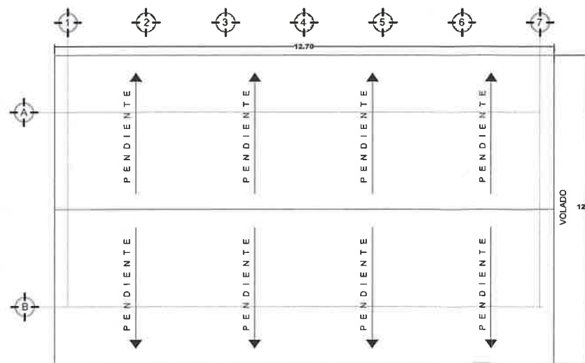
PLANTA DE AZOTEA TALLER DE ELECTRICIDAD ESC. 1:100
