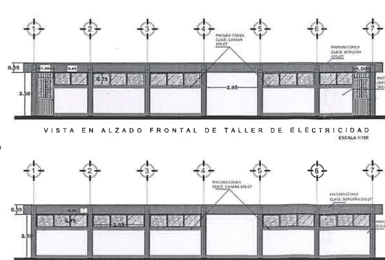
VISTA EN ALZADO POSTERIOR DE TALLER DE ELECTRICIDAD ESCALA 1:100
