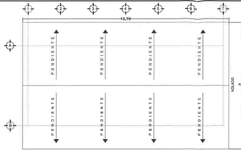
PLANTA DE AZOTEA TALLER DE CARPINTERÍA ESC. 1:100
