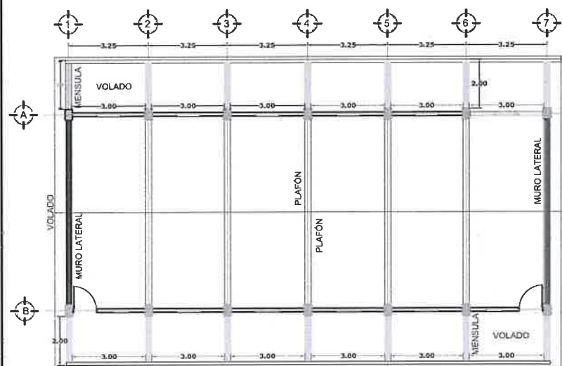
VISTA EN PLANTA TALLER DE ELECTRICIDAD ESC. 1:100
