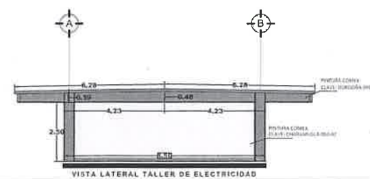
VISTA LATERAL TALLER DE ELECTRICIDAD
