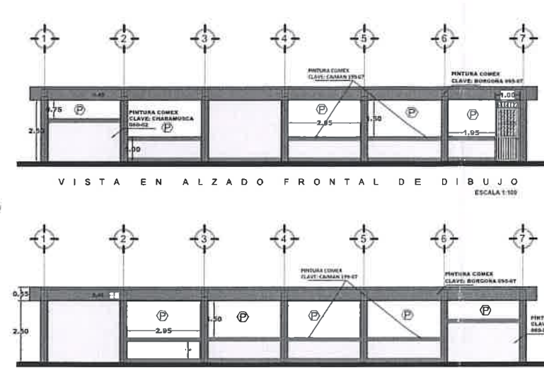
VISTA EN ALZADO POSTERIOR DE DIBUJO ESCALA 1:100
