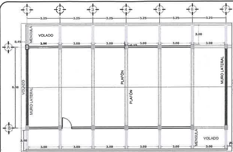
VISTA EN PLANTA TALLER DE CARPINTERÍA ESC. 1:100
