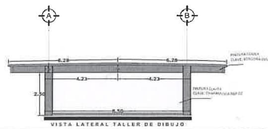
VISTA LATERAL TALLER DE DIBUJO
