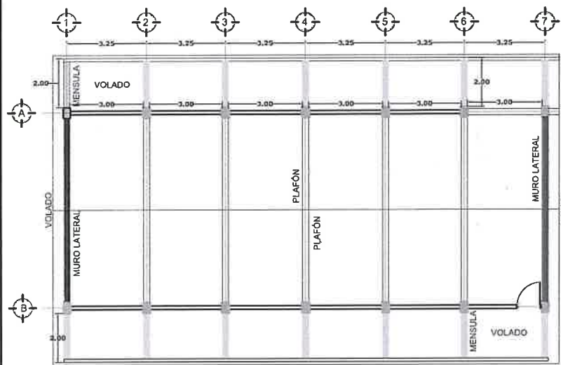
VISTA EN PLANTA TALLER DE DIBUJO ESC. 1:100
