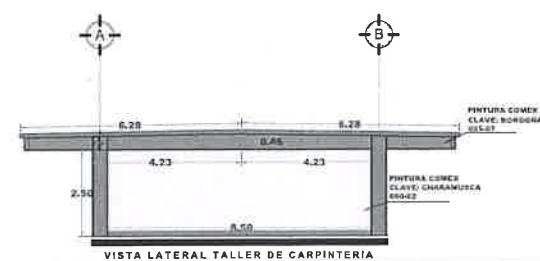
VISTA LATERAL TALLER DE CARPINTERÍA
