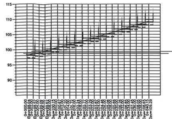
PERFIL LADO ESTE ESCALA HORIZONTAL 1 : 1000 ESCALA VERTICAL 1 : 1000
