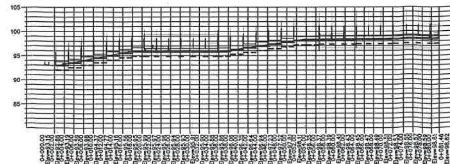
PERFIL LADO OESTE ESCALA HORIZONTAL 1 : 1000 ESCALA VERTICAL 1 : 1000
