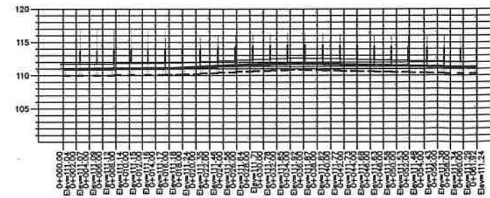
PERFIL LADO SUR 2 ESCALA HORIZONTAL 1 : 1000 ESCALA VERTICAL 1 : 1000
