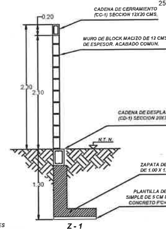
CORTE A-A' ALZADO TIPO 1
