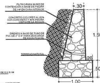
ALZADO DE MURO CICLOPEO
