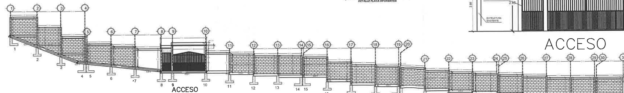
PERFIL LADO NOROESTE
