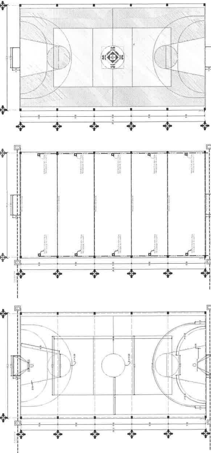
DISEÑO CANCHA PINTURA DEPORTIVA ESC. 1:100
