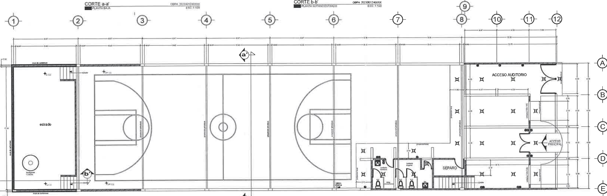
PLANTA ARQUITECTÓNICA PLANTA BAJA ESTRADO OBRA: 2023301240191 ESC: 1:100
