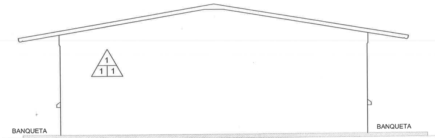
FACHADA LATERAL ESC. 1:75 ACABADOS
