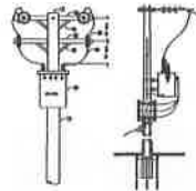
TRANSFORMADOR 10 KVA
