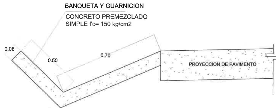
DETALLE DE CUNETA
