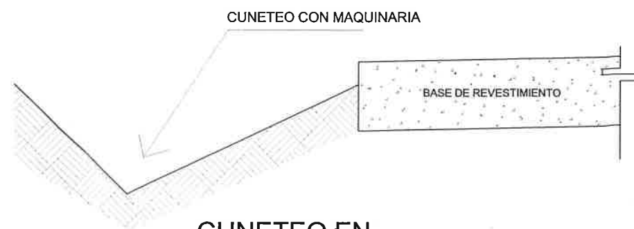
CUNETEO EN REHABILITACION DE CAMINO
