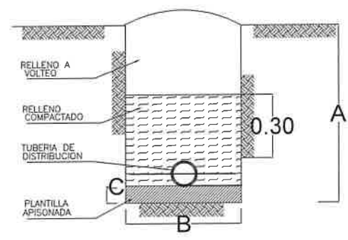
SECCION DE ZANJA
